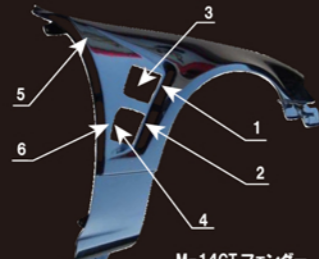
M-14GT フェンダーダクト付・網付車 ※穴あけ指定場所番号
